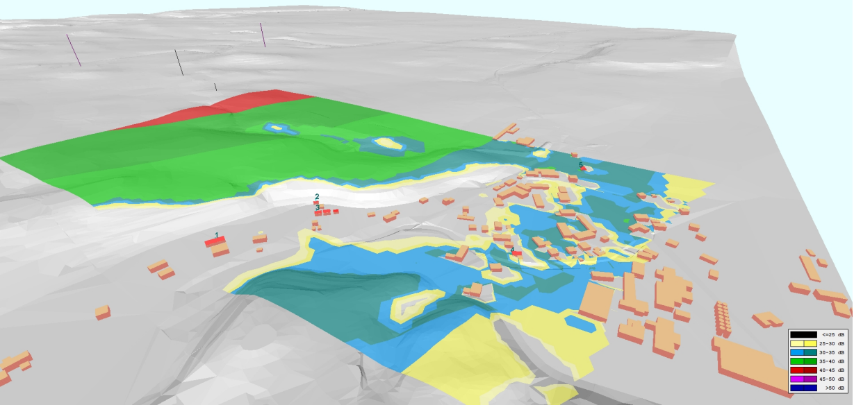
Příloha č. 6. STAV 1 detail 3D, výška pásem izofon 3 m n.t.
